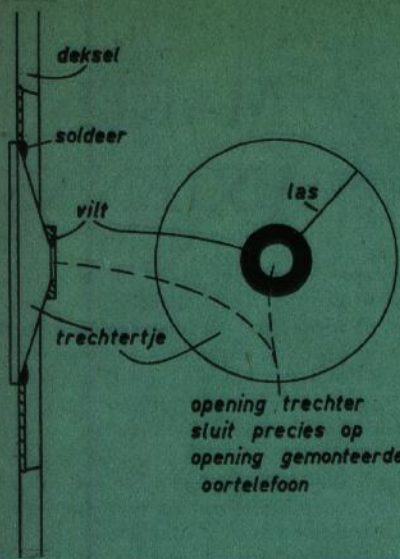
.... trechtertje in doosdeksel
